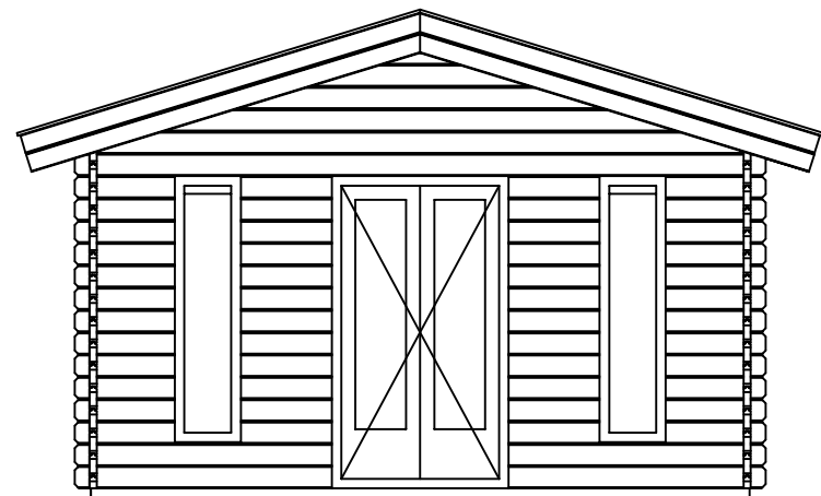
vooraanzicht / front view / vorderansicht
